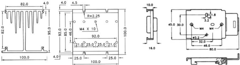
TSR-100 или HS-100: Радиаторы для трехфазных реле
